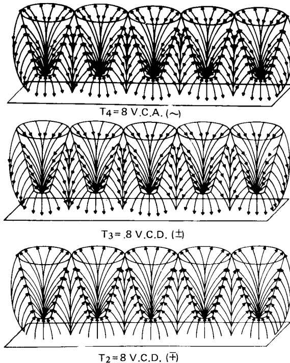
Figura 2. Forma aproximada de las líneas de campo eléctrico, para cada uno de los tratamientos eléctricos T 2 , T 3 y T 4 para un instante de tiempo.
